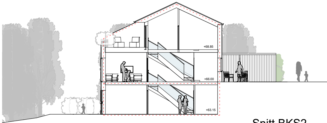
Snitt BKS2 1 : 200
