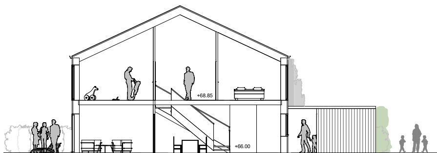
Snitt BKS1 1 : 200
