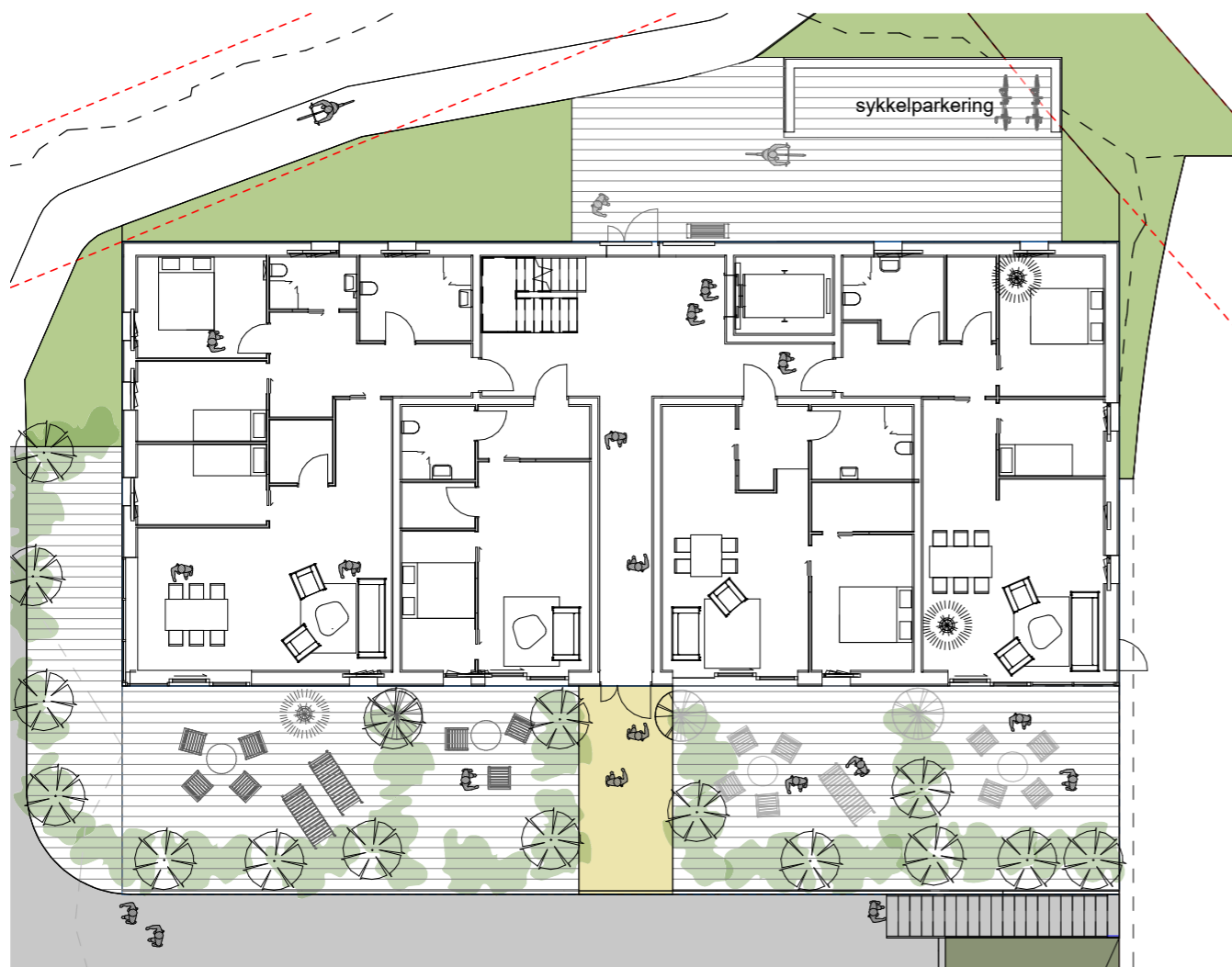
Plan BBB3 - 01 etasje 1 : 200
