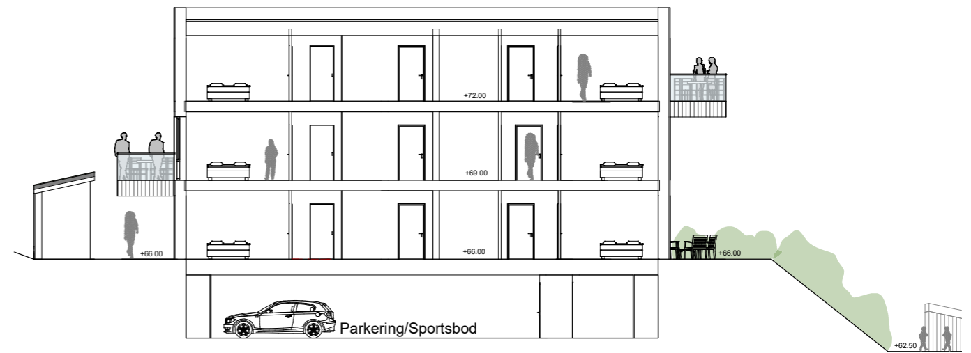
Snitt BBB1 - bb 1 : 200
